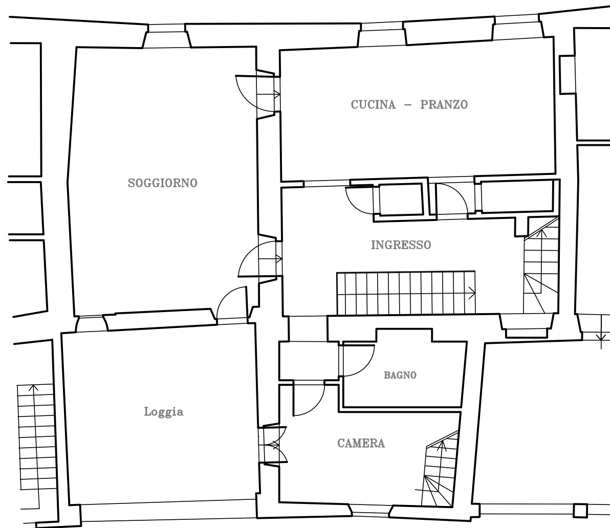
PIANO PRIMO SCALA 1:100
